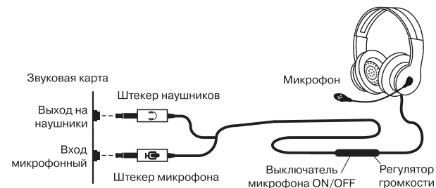
Рис. 1. Схема подключения
